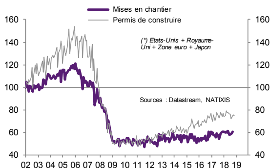
Graphique 11a OCDE* : mises en chantier et permis de construire (100 en 2002:1)
