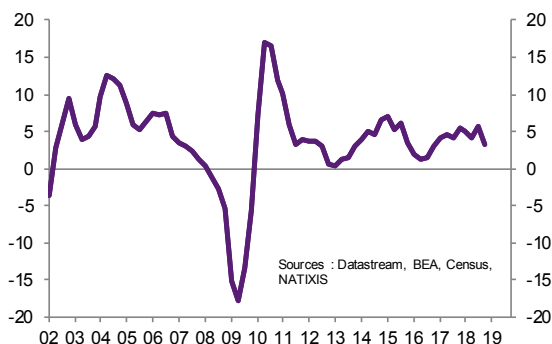
Graphique 7 Etats-Unis : importations (volume, GA en %)
