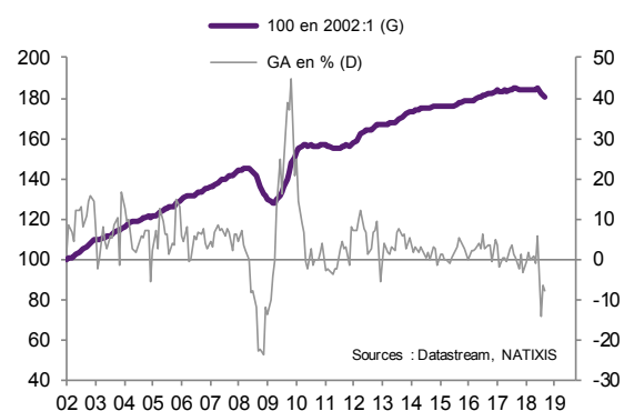
Graphique 10 Monde : ventes de voitures
