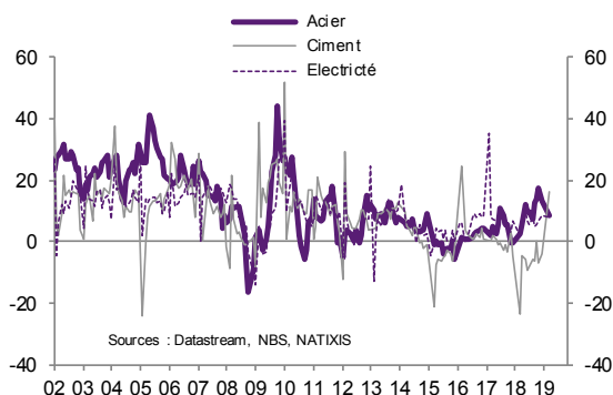
Graphique 13a Chine : production (GA en %)
