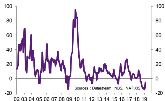
Graphique 13b Chine : production (GA en %)
