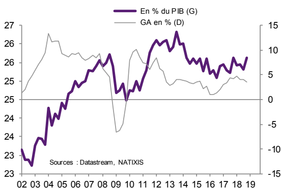
Graphique 9 Monde : investissement volume
