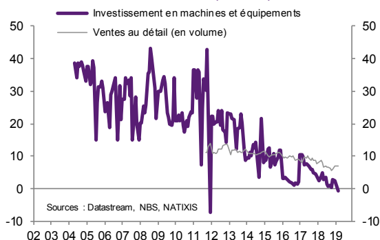
Graphique 12a Chine : investissement en machines et équipements et ventes au détail (GA en %)
