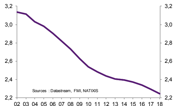
Graphique 8 Royaume-Uni : PIB en $PPA (en % du PIB Monde en $ PPA)
