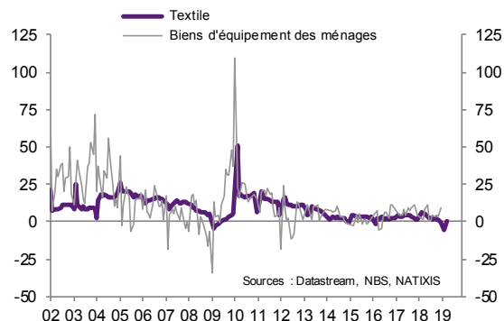
Graphique 13b Chine : production (GA en %)
