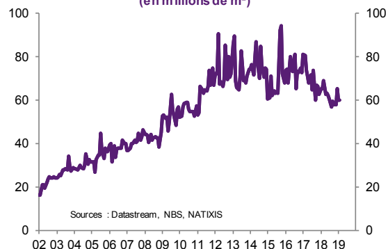
Graphique 11b Chine : construction - logements terminés (en millions de m 2 )
